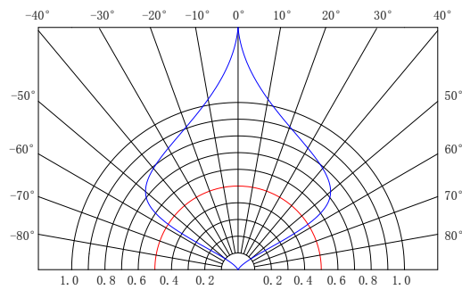
Lighting Angle / 發光角度：
