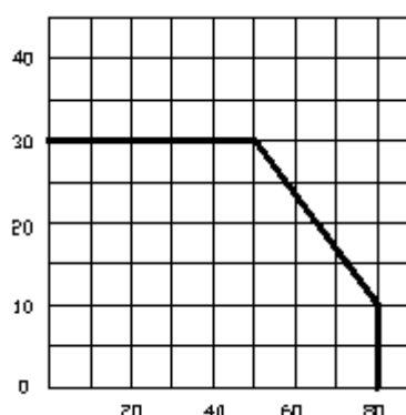
Maximum Forward Current vs. Ambient Temperature 環境溫度與電流的關係
