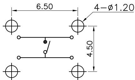
PCB Layout(Pattern Side)
